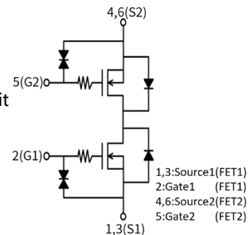
原理图 Schematic diagram
